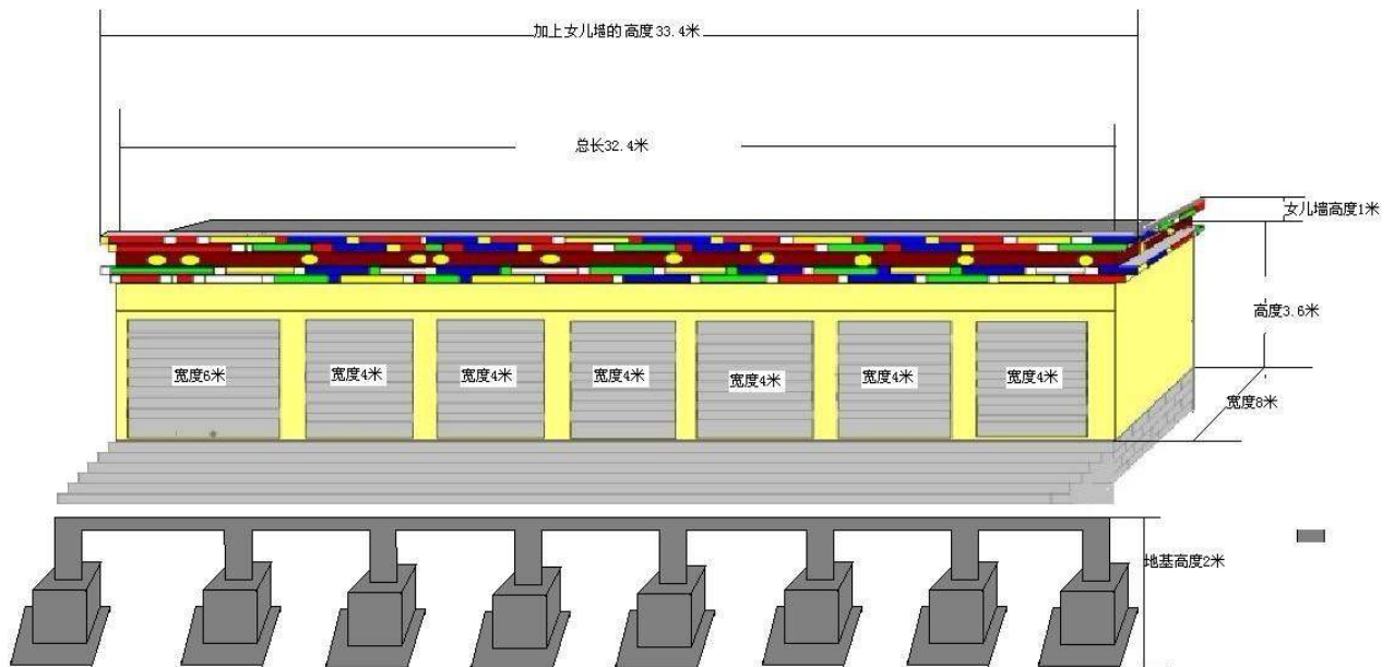
-- tekening van het fundament (op palen en blokken) --
